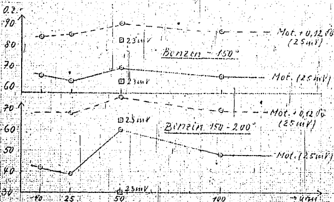
Abb. 5: Oktananzahlen der Benzine
