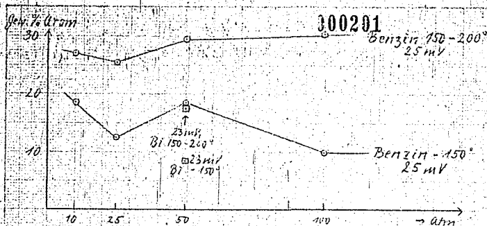
Abb. 3: Gew. % Aromaten im Benzin
