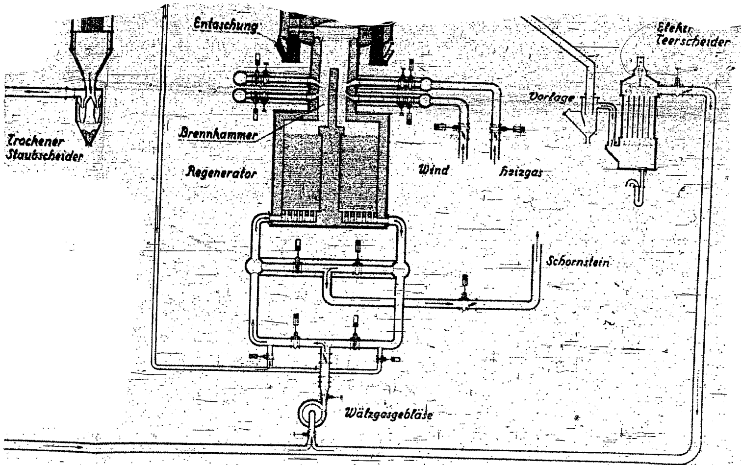
Schema der Pintsch-Hütte- brand Wassergasanlage
